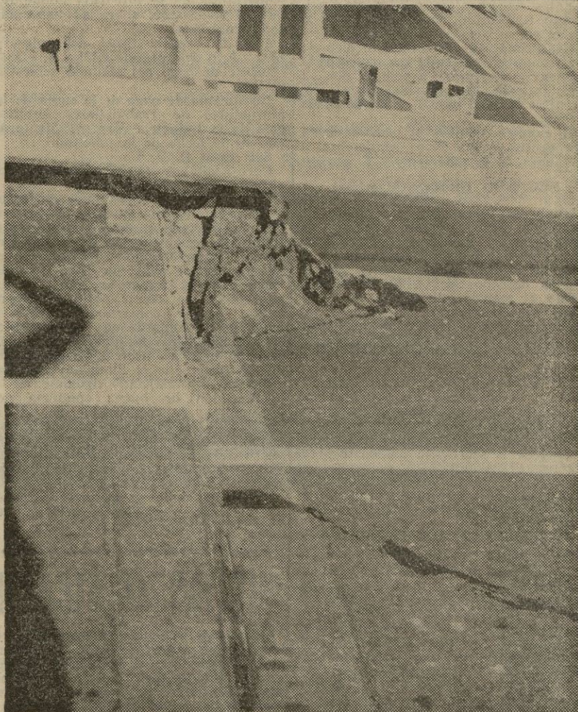
Dos vistas de cómo quedó el puente en su parte alta. En una de ellas se aprecia detalladamente la grieta que se produjo en el asfalto, y en la otra se da una visión del descenso de nivel que experimenta el firme en su parte central. Desde las doce y cuarto hasta las seis de la tarde, el nivel del puente, en las vigas destrozadas, había bajado más de medio metro.
