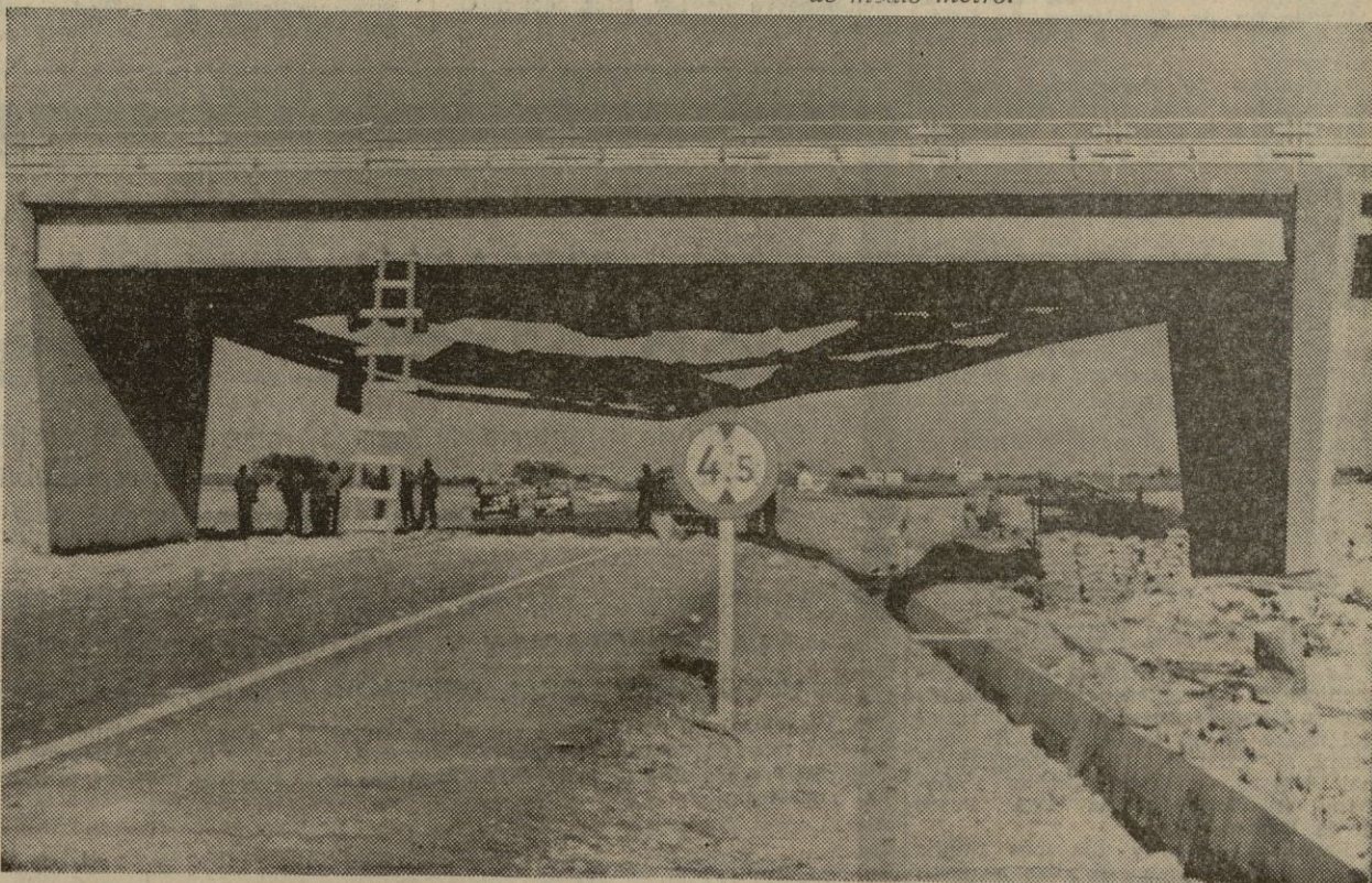
La señal está claramente colocada a veintiséis metros del puente, por los dos lados. El conductor del camión admite que la vio, pero no la respetó. «Ya había pasado otros puentes antes y no había pasado nada».
