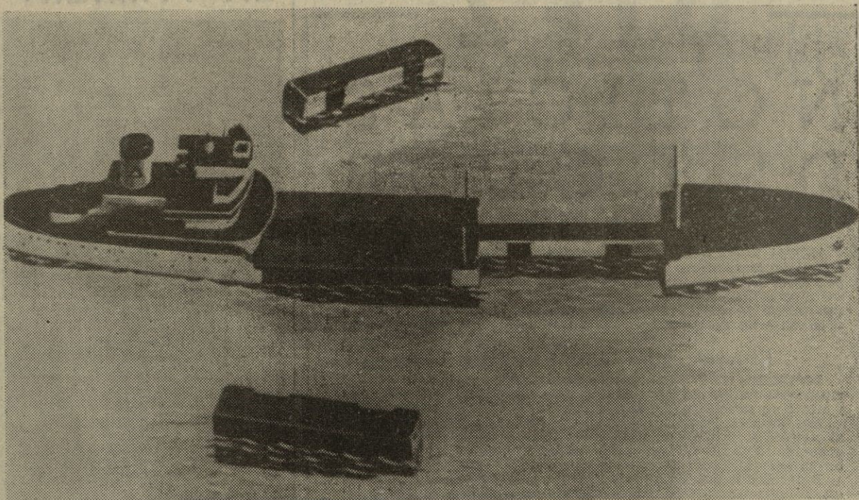
El armador de barcos Onassis tiene en proyecto la construcción de un nuevo tipo de petrolero que lleva cuatro tanques independientes que se pueden colocar o separar del buque, según las necesidades de carga. La capacidad es de un millón de toneladas y tendrá más de 500 metros de largo por 85 de ancho con una profundidad de 47 metros. — (Telefoto AP-EUROPA PRESS)
