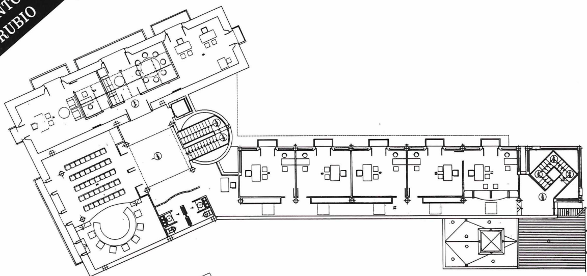
Planta primera
