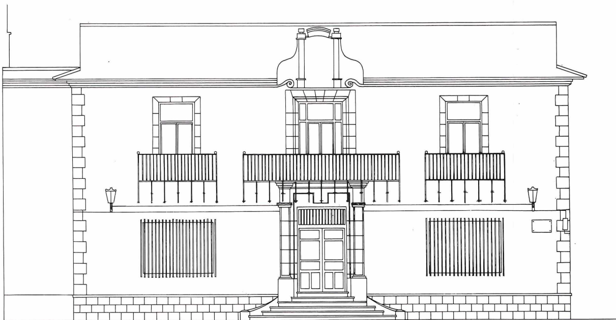
Alzado de la fachada frontal a la plaza de la Encarnación. Situación actual.
