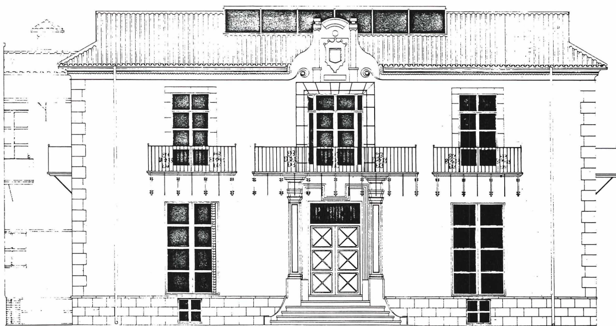
Alzado de la fachada frontal a la plaza de la Encarnación. Propuesta.
