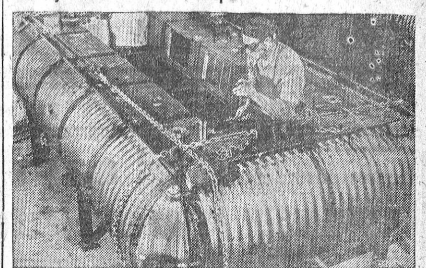
Un soldador montando las secciones completas de una nueva lancha salvavidas destinada a los barcos mercantes, en una fábrica de los E.E. U.U. La lancha tiene cabida para veinte hombres, contiene una estufa de carbón vegetal para cocinar y calentarse, agua y viveres para un mes, una caperuza de protección contra la lluvia y el viento y cojines impermeables, además de otros artículos. — (Foto WHITE.)
