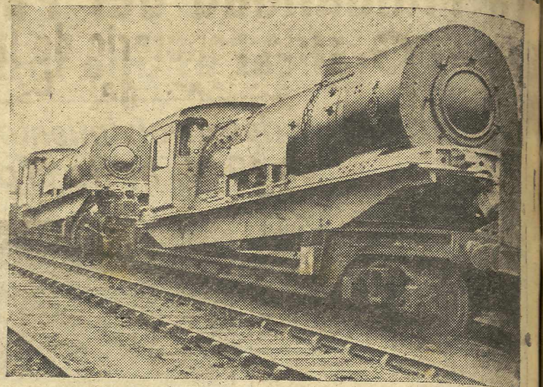
Las dos primeras locomotoras Bayer-Garratt de 184 toneladas, de un peso neto de 20, para los ferrocarriles de Rhodesia, a su salida de Manchester para el puerto de embarque.
